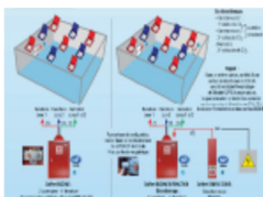
Bâtiment supérieur à 500 m2 + coffret 2O/F TYPE CONFORT
